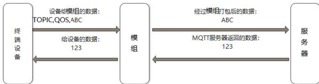
图 6 MQTT 模式通信示意图
