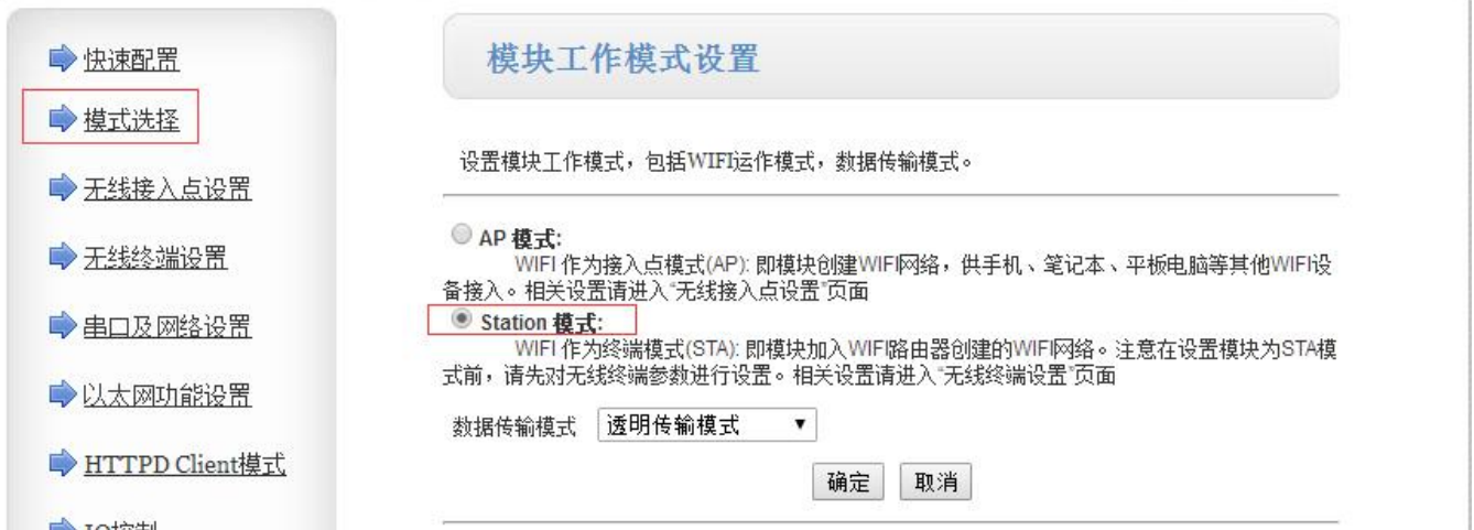
图 3 网页方式设置 WIFI 模式
