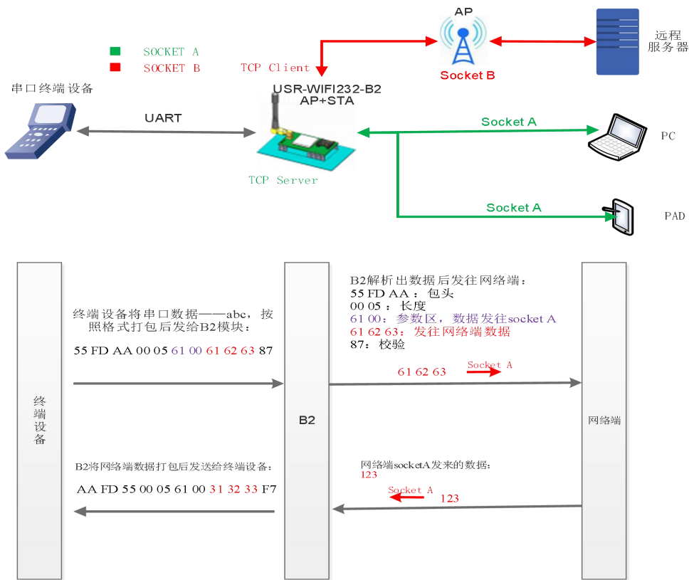
图 36 套接字分发框图
