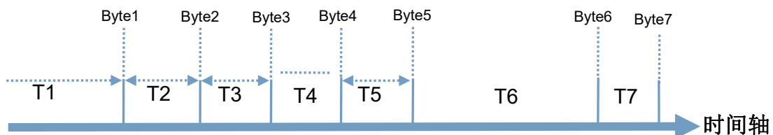
图 20 切换指令模式时序
