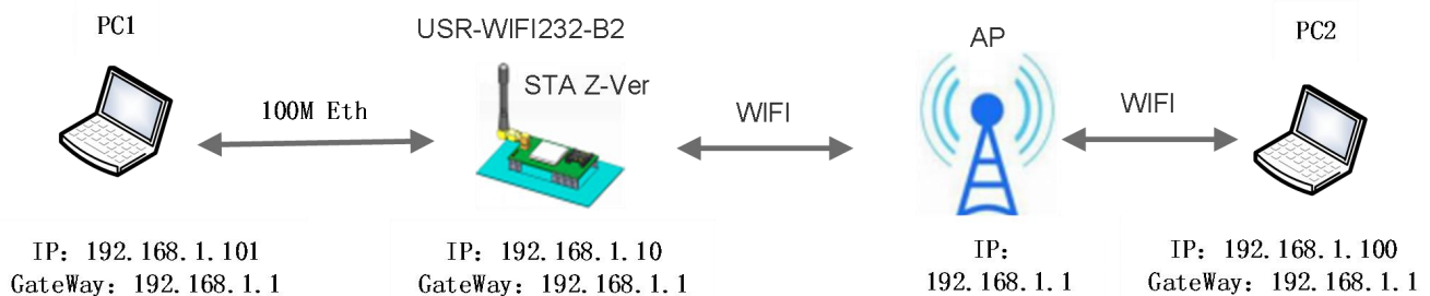
图 11 USR-WIFI232-B2 以太网接口功能（STA Z-Ver）
