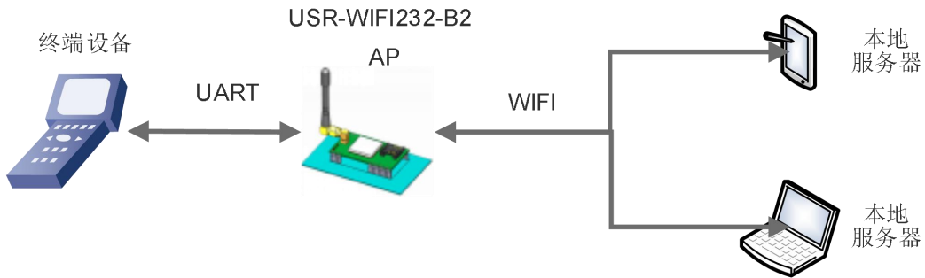
图 5 USR-WIFI232-B2 自组网 1
