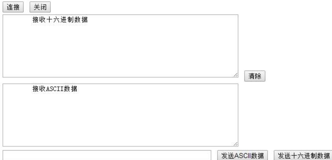
图 48 WebSocket 页面
