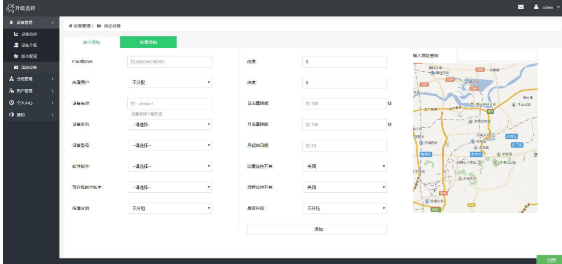
图 33 添加设备
