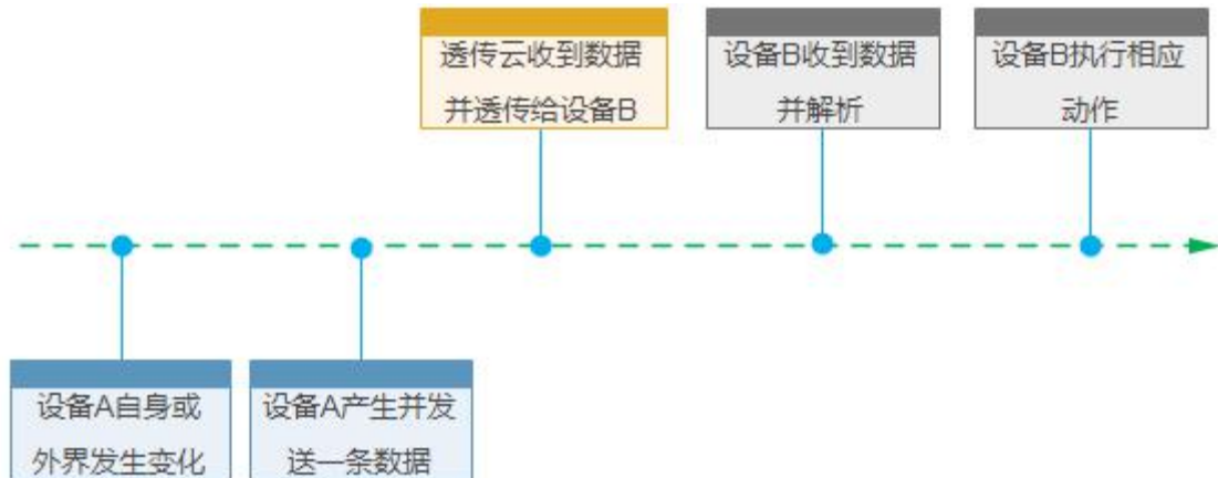
图 24 数据转发流程
