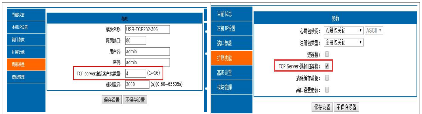
图 38. TCP Server 连接 Client 最大值与踢掉旧连接设置
