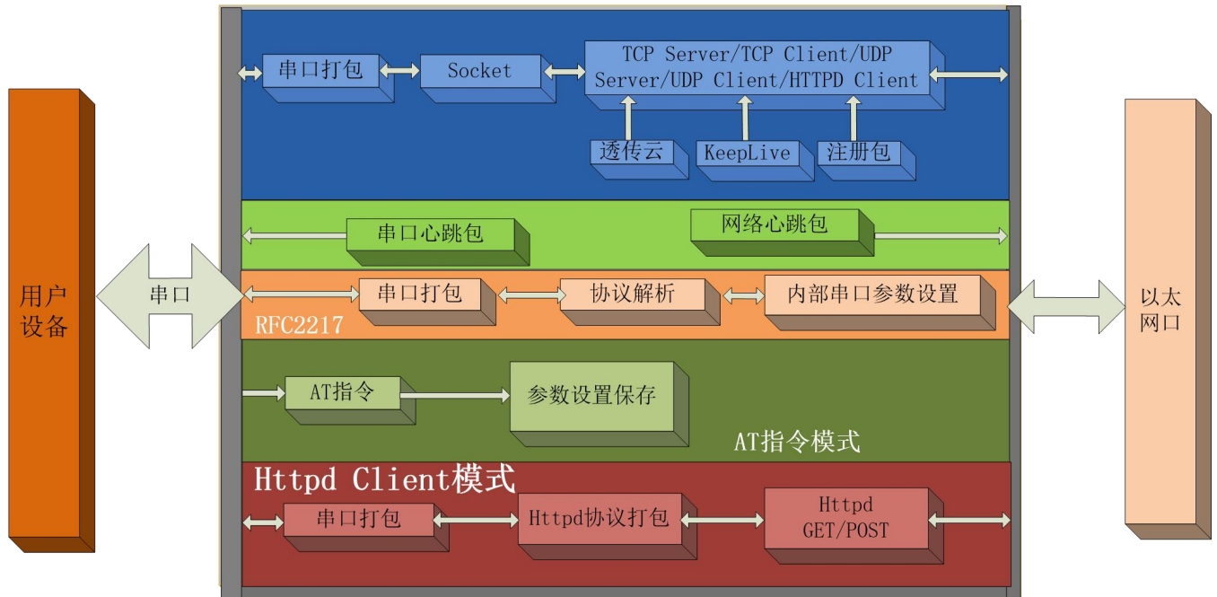
图 1. 306 功能框图
