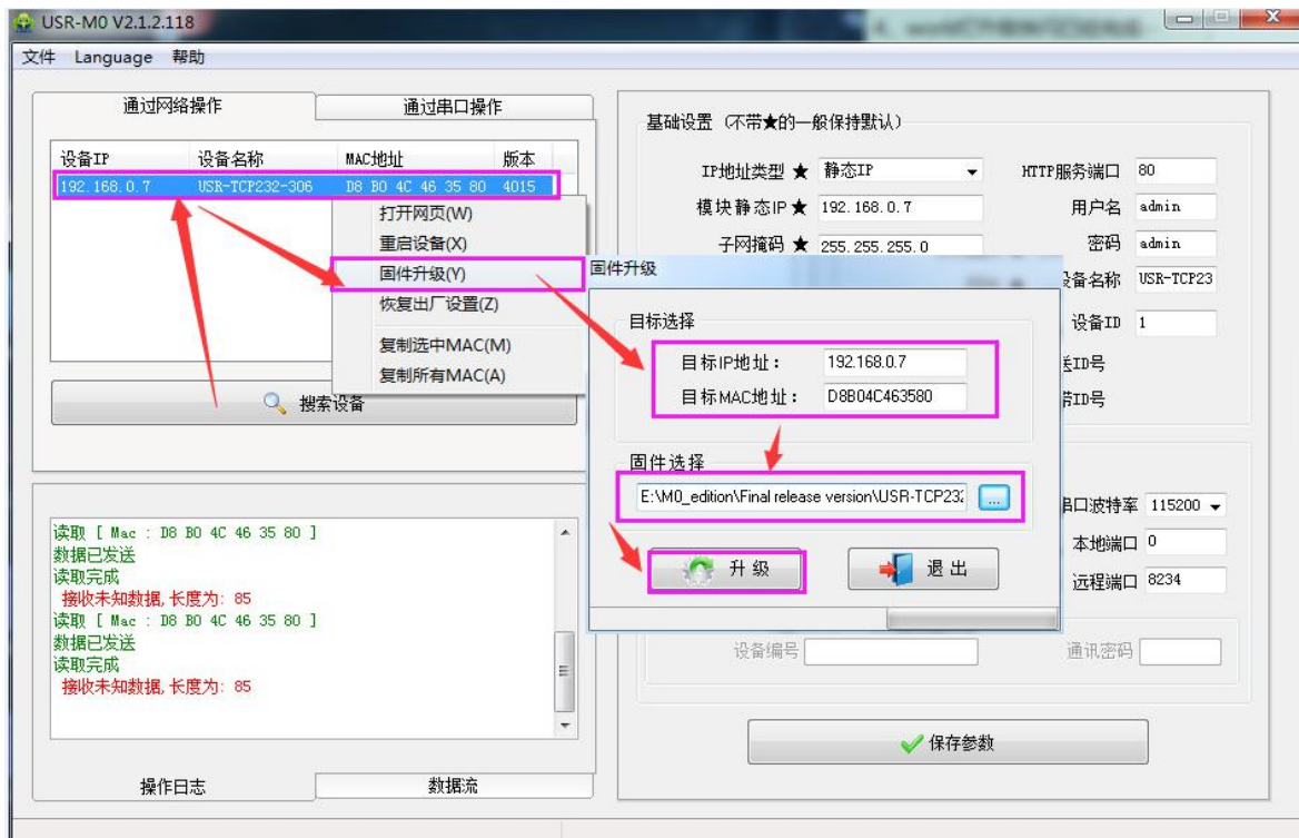
图 5. 选择固件
