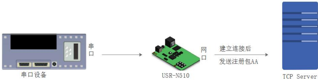
图50 注册包建立连接发送注册包
