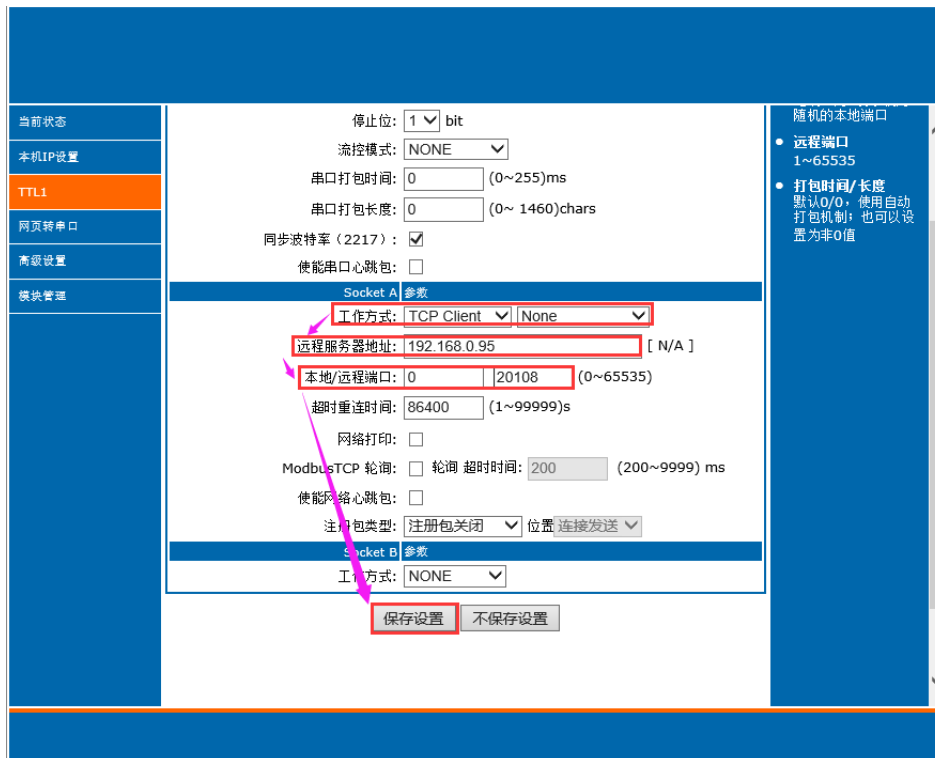
图10 TCP Client 网页设置
