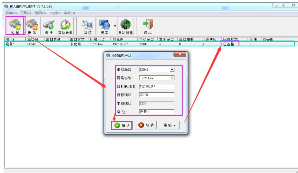
图31 VCOM 应用模式添加串口
