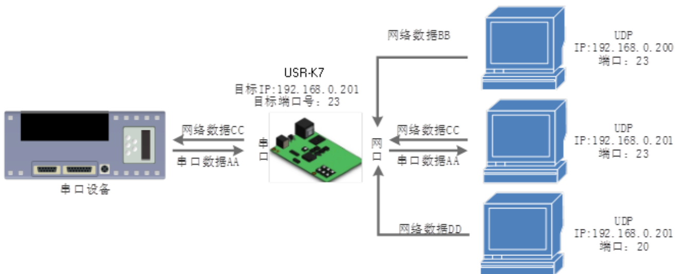
图16 UDP Client 模式说明
