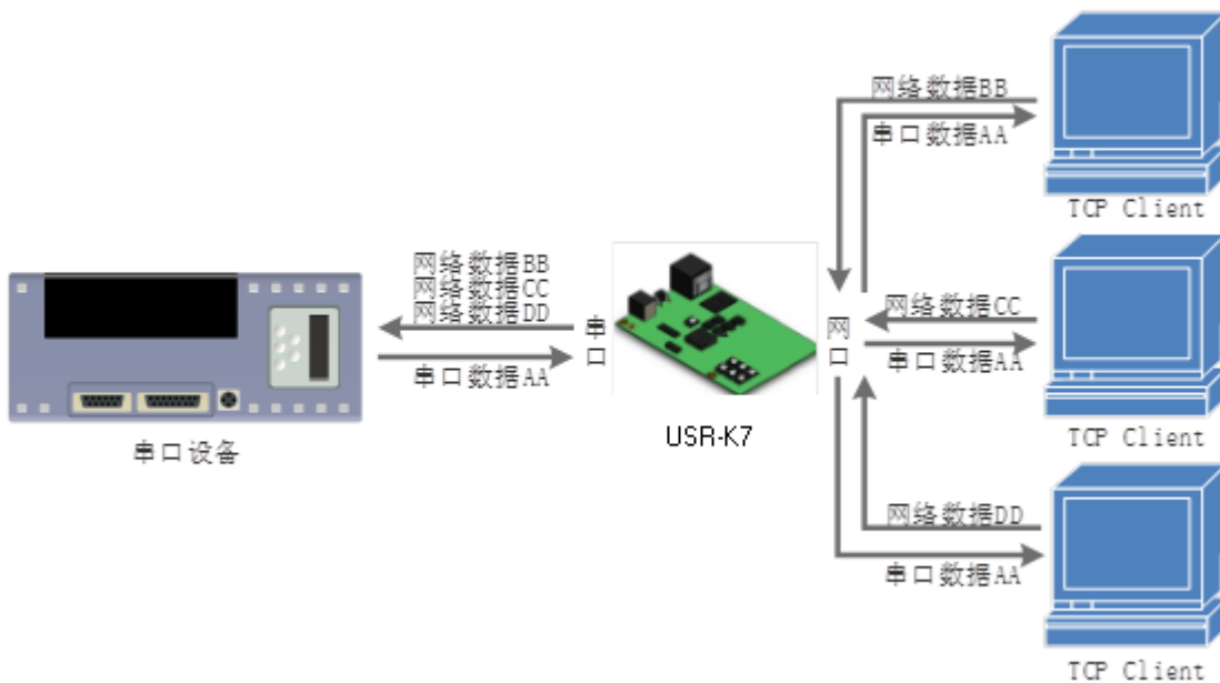
图12 TCP Server 模式说明
