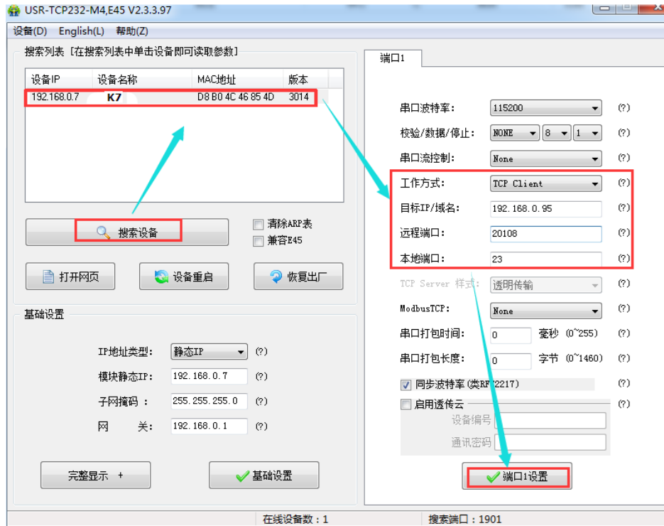
图9 TCP Client 软件设置
