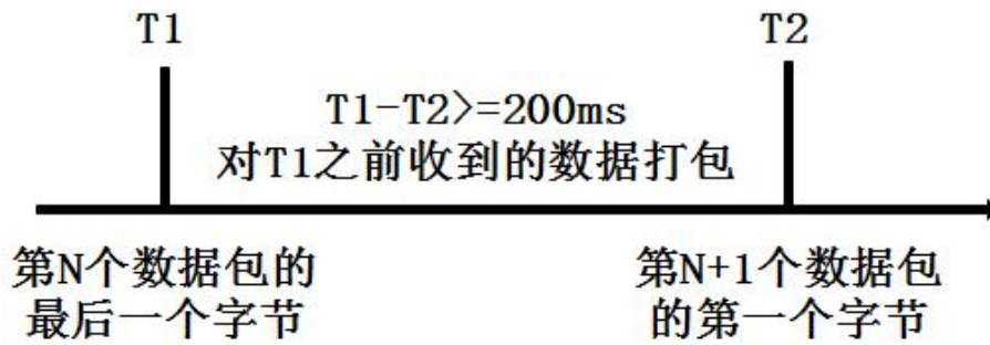
图 9 成帧机制示意图
