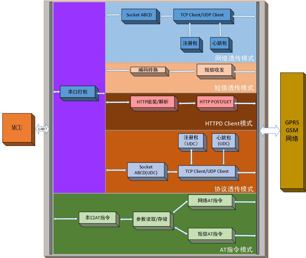
图 1 功能框图
