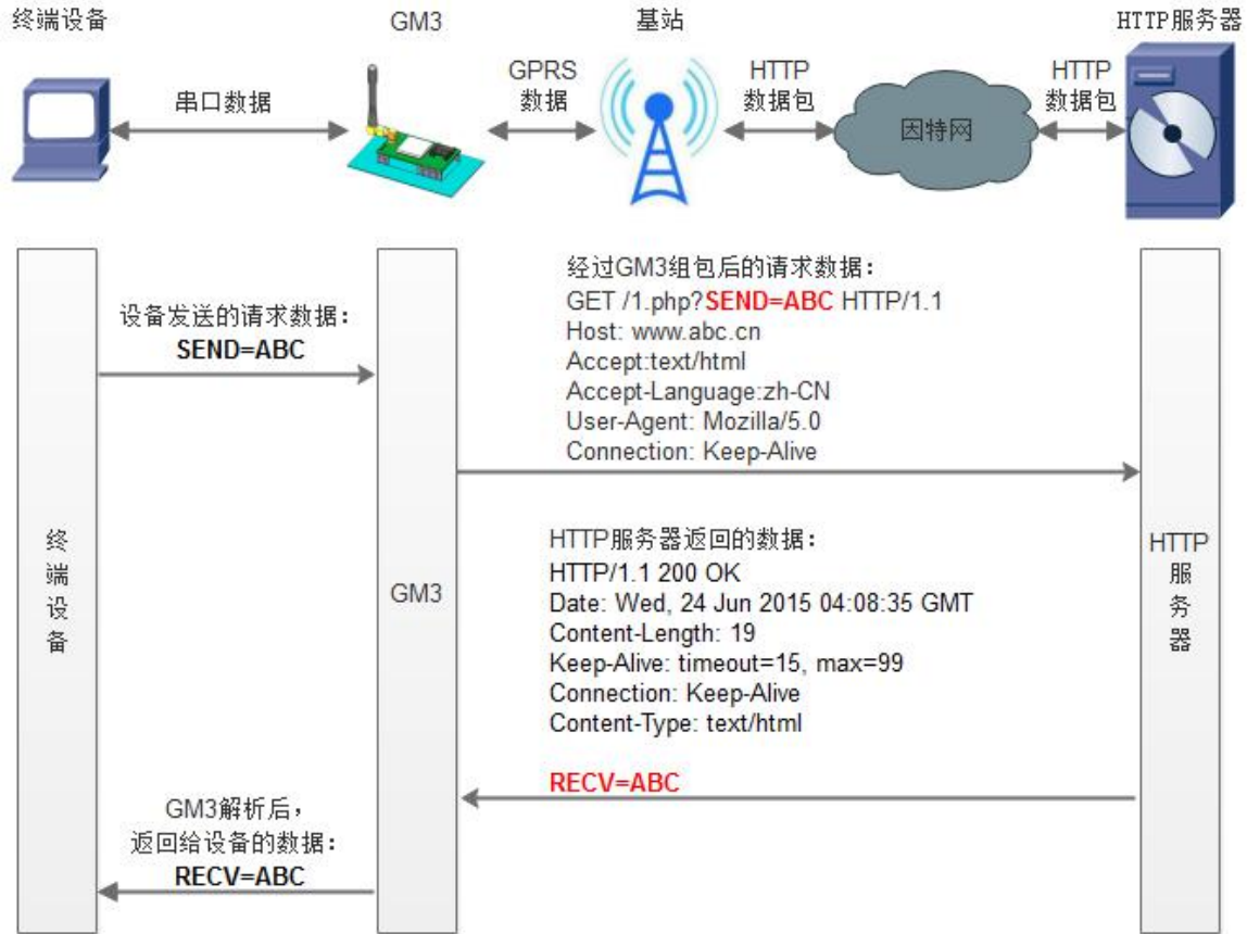
图 4 HTTPD 模式
