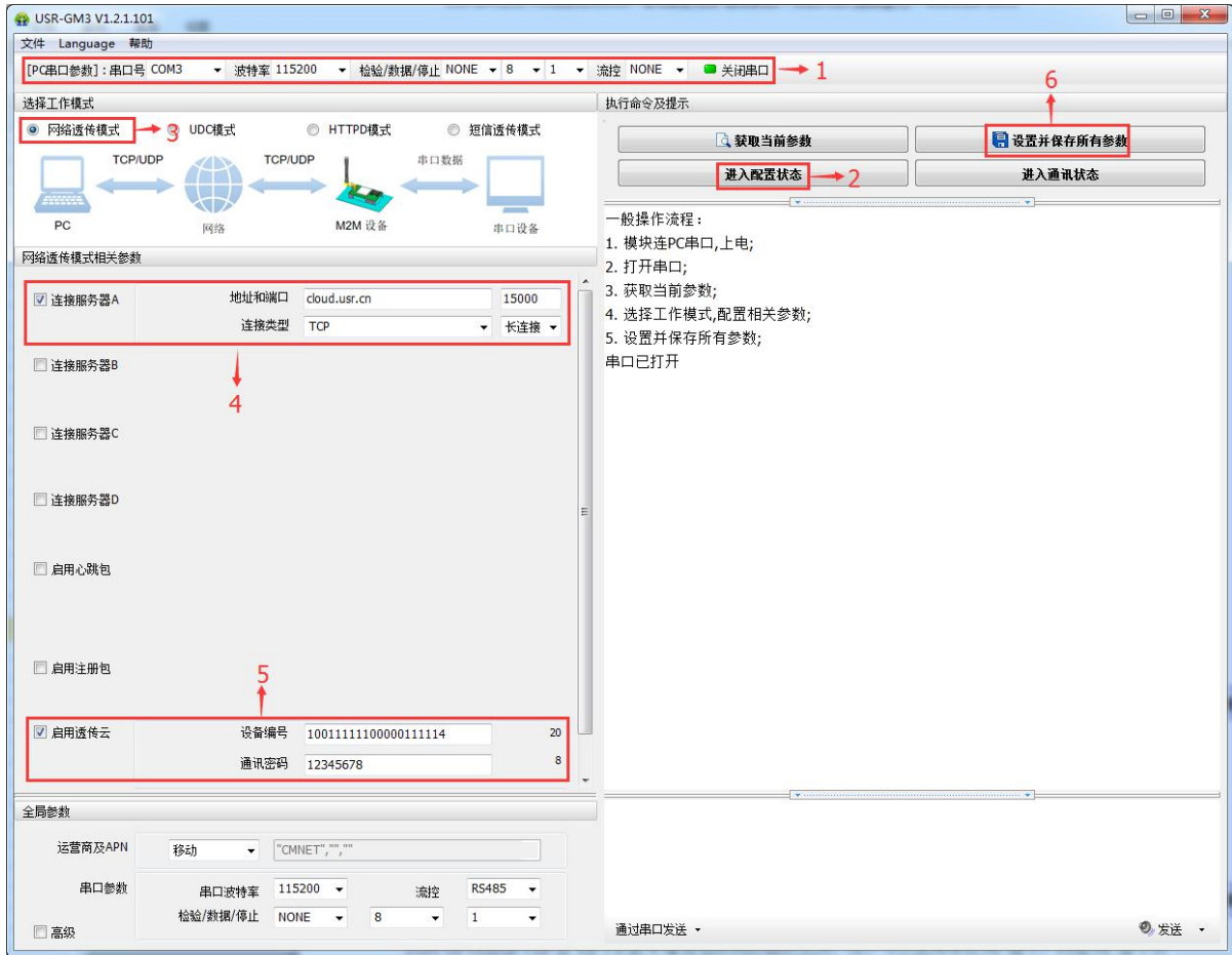
图 16 设置软件示意图
