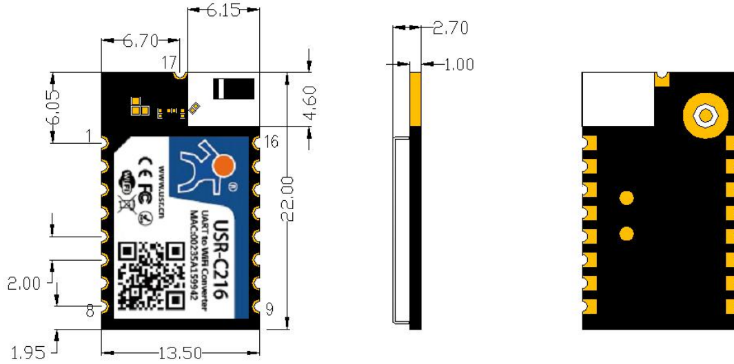
图 6 USR-C216 尺寸图
