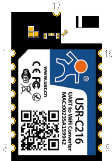
图 7 USR-C216 引脚图
