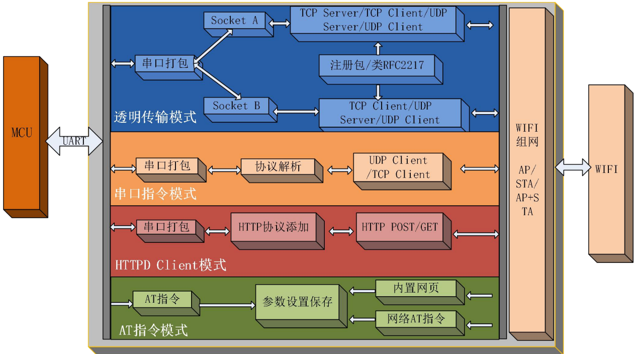
图 8 功能框图
