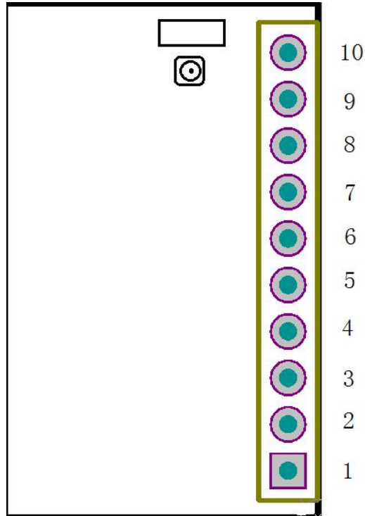
图 8 USR-C215 引脚图
