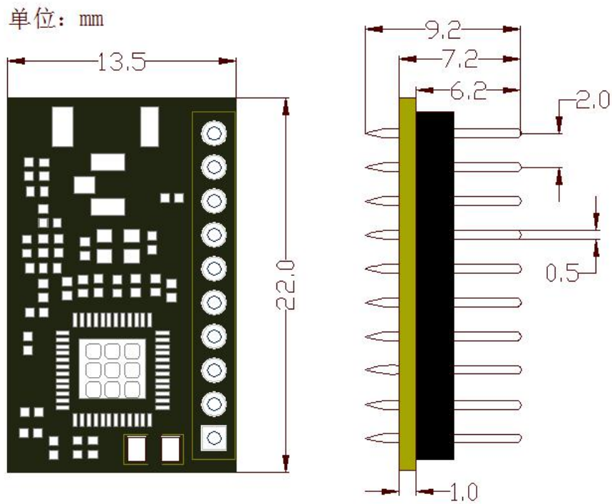
图 7 USR-C215 尺寸图
